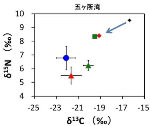
図4 五ヶ所湾と生浦湾のアサリと懸濁態有機物(POM)と堆積物(SOM)の安定同位体比 C-N マップ
